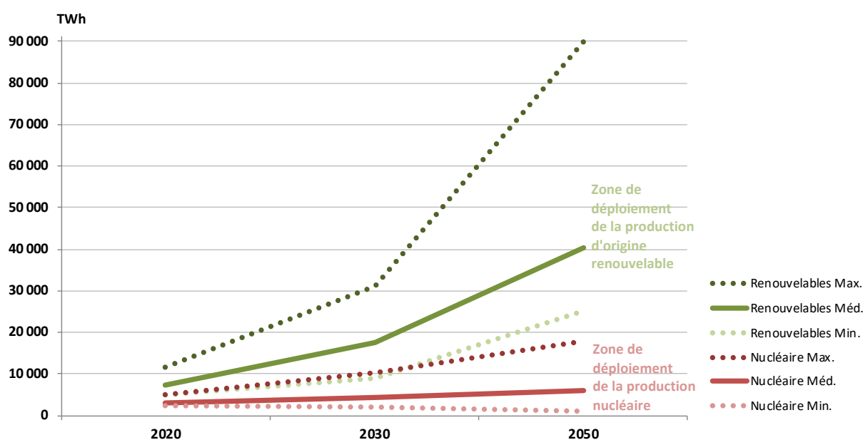
Figure 12 – Trajectoire minimum, médiane et maximum de production d'électricité d'origine renouvelable et de production d'électricité nucléaire en 2030 et en 2050 dans l'ensemble des trajectoires 1,5°C sans dépassement ou avec dépassement minimale (50 trajectoires) Source : Association négaWatt (2020), d'après GIEC (2018)
